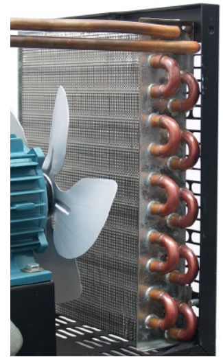
Refrigeración mediante doble serpentín para una refrigeración optimizada.
